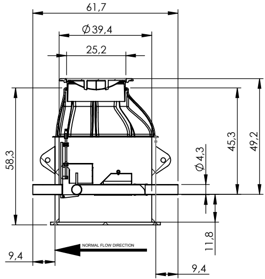
A-A SCALE 1 : 40
