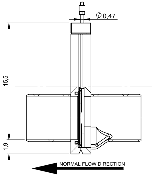
A-A SCALE 1 : 7.5
