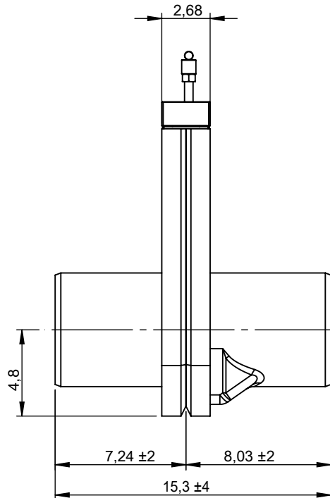
A-A SCALE 1 : 7.5
