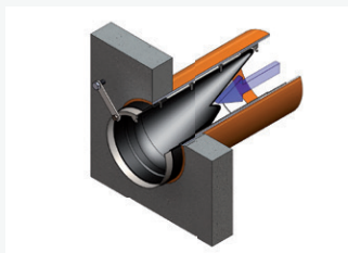
KAMMERINSTALLATION
